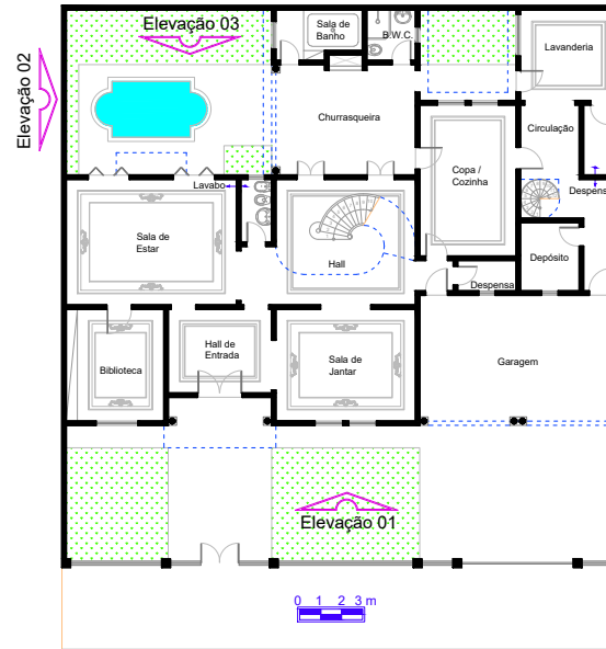
Térreo A = 242,89 m 2
