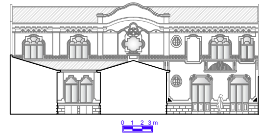
Elevação 03
