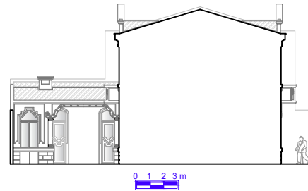
Elevação 02
