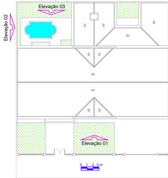
Implantação e Cobertura
