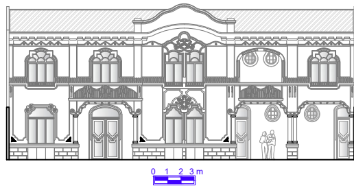
Elevação 01
